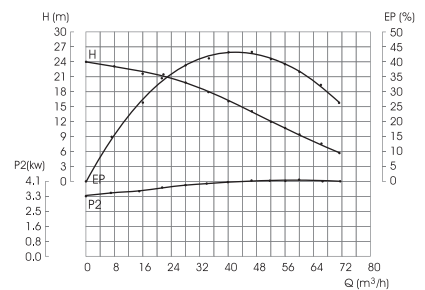
KDP40/KGP40 //: Performanțe
