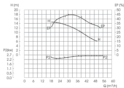
KDP30/KGP30 //: Performanțe
