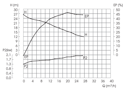
KDP20/KGP20 //: Performanțe
